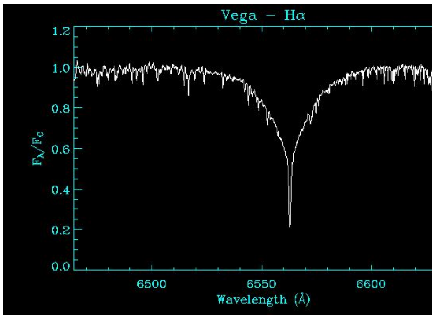
H-alpha region
