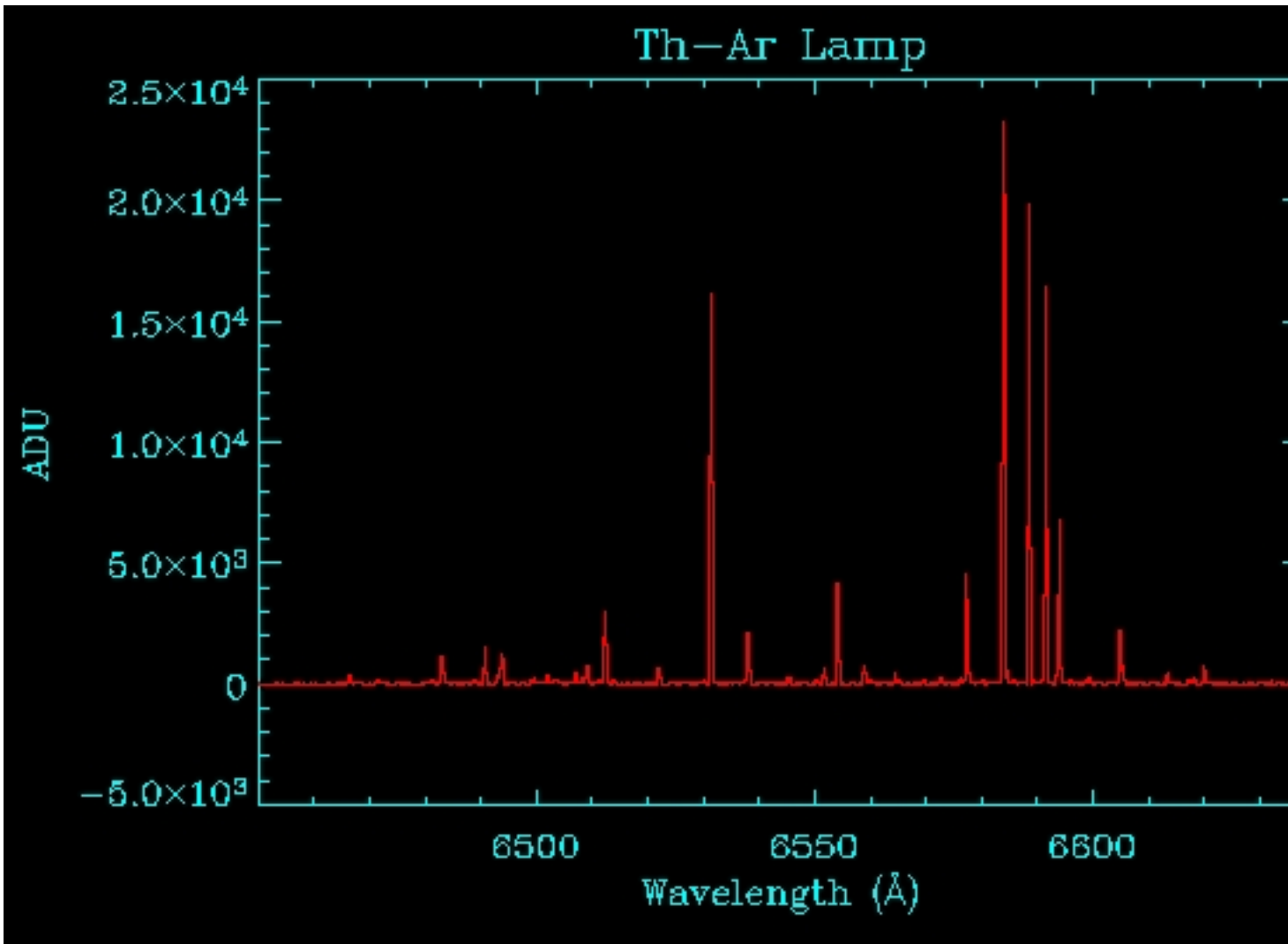
H-alpha region
