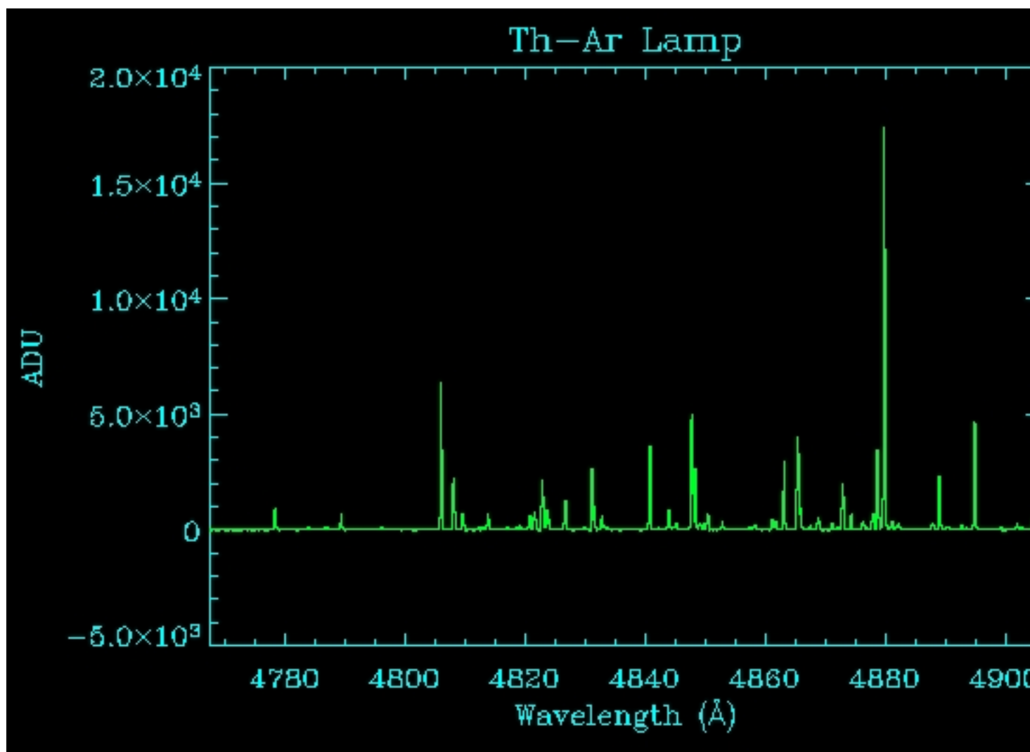
H-beta region
